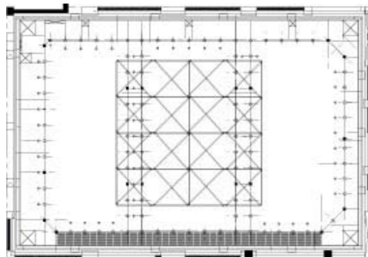
PIANTA DELLA SALA CON LA STRUTTURA METALLICA / ROOM PLAN SHOWING THE METAL STRUCTURE
